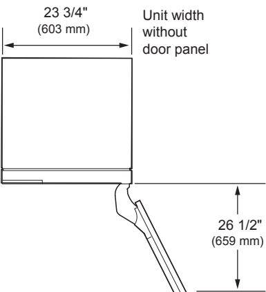
DOOR OPEN 115°
