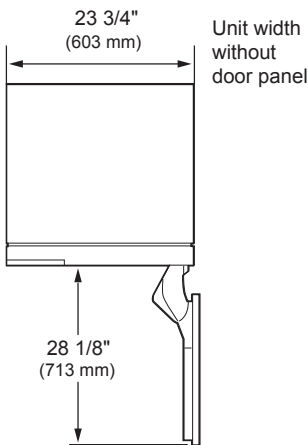
DOOR OPEN 90°
