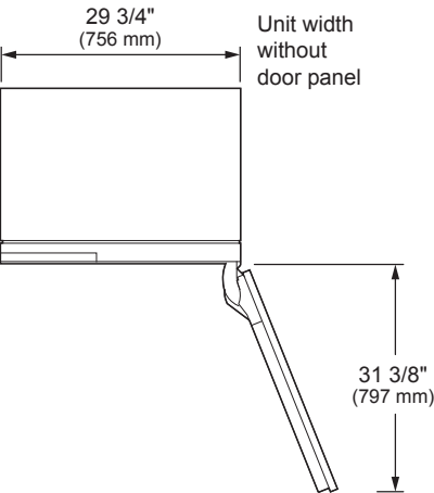
DOOR OPEN 115°
