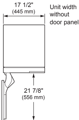
DOOR OPEN 90°
