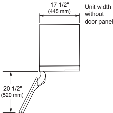
DOOR OPEN 115°
